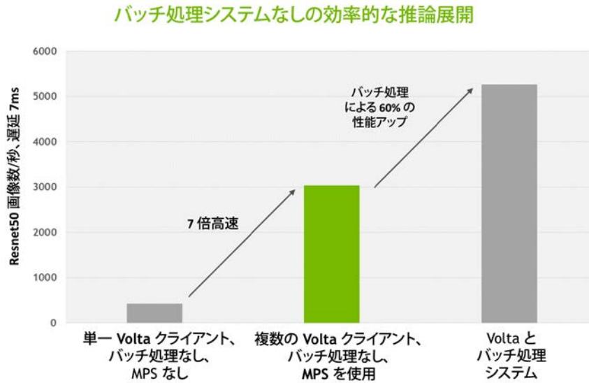
図 26. Volta MPS による推論
