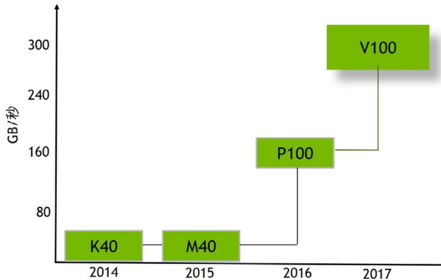
図 14. 第 2 世代 NVLink のパフォーマンス
