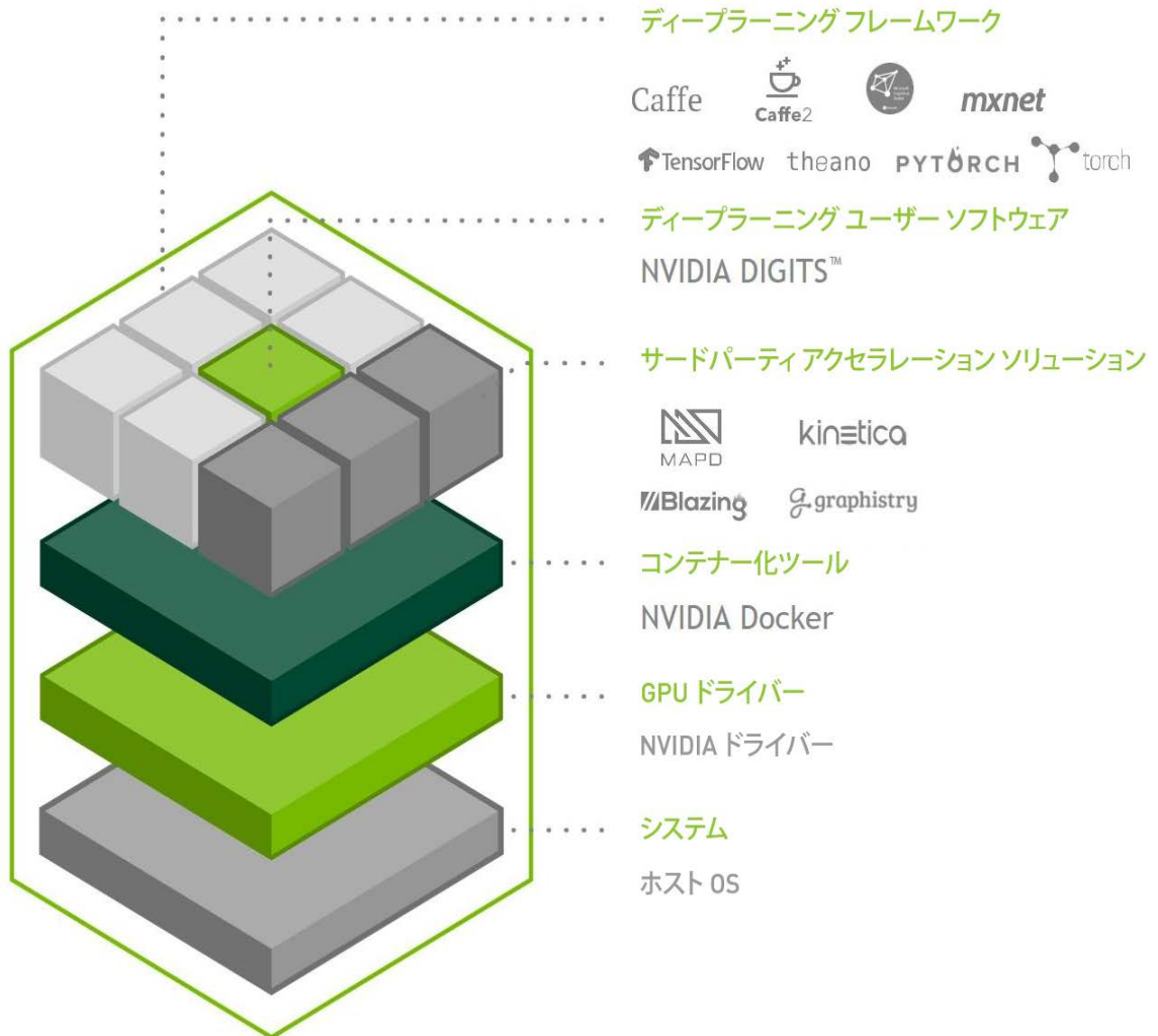
図 30. 生産性を瞬時に向上できる完全統合型の NVIDIA DGX-1 ソフトウェアスタック
